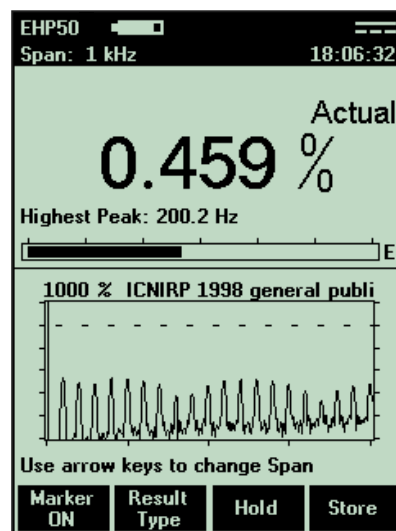
标准模式显示被测场强的频谱并根据 ICNIRP 准则对其进行评估，图中虚线表示限值 (100%)
